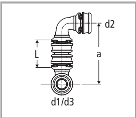
Optiflex-Flowpress-T-Stück mit Optiflex-Flowpress-Bogen 90° 84242/84240
